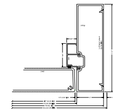
2650 LOCK JAMB
