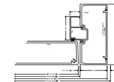
2450 LOCK JAMB
